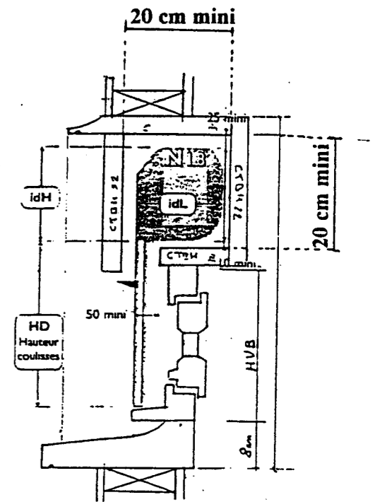
Coupe verticale d'un volet roulant
