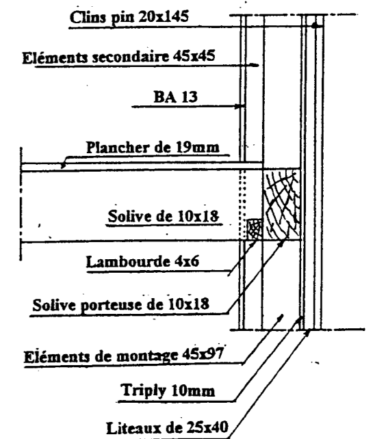
Détail du solivage dans le mur d'ossature bois
