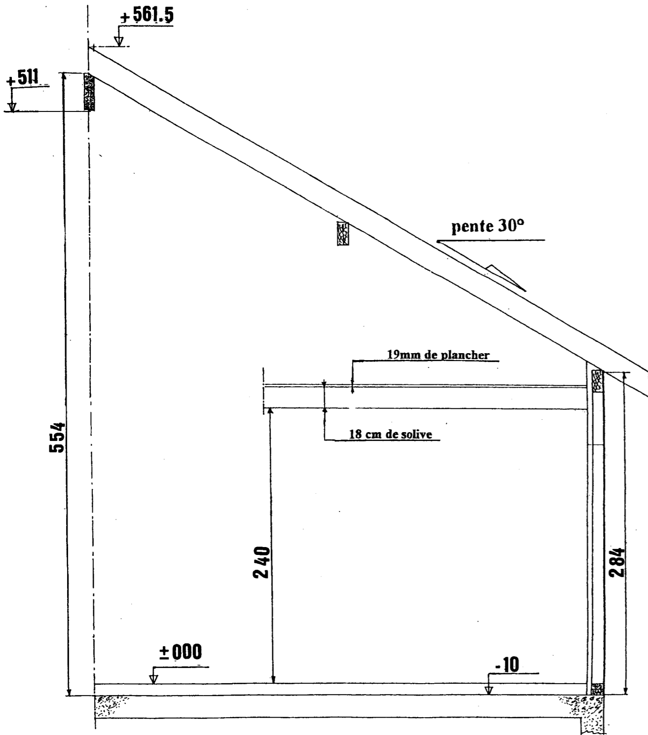
Coupe verticale A-A
